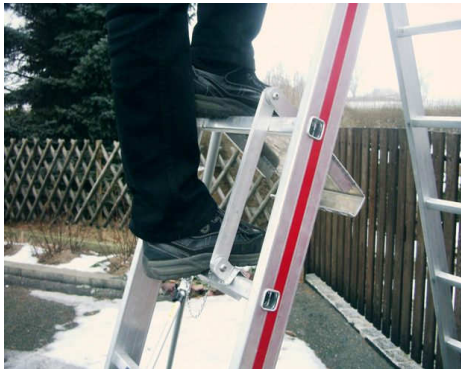
Bild 1: Einhängevorrichtung eingeklappt
