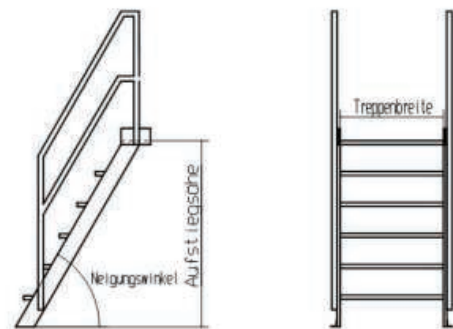
Treppenzugang, stationär
