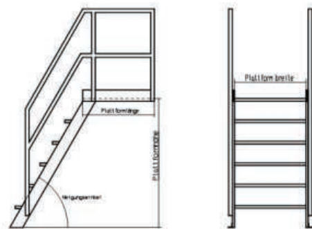
Podesttreppe, stationär
