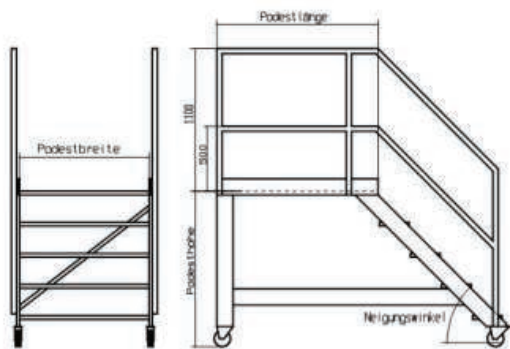
Podesttreppe mit Plattform, fahrbar
